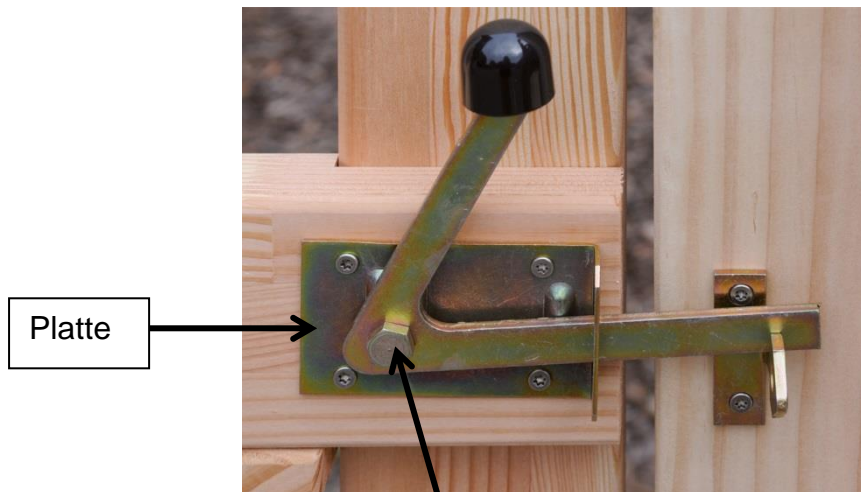
Diese Schraube lösen um Klinkhaken zu drehen.
