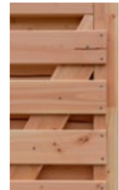
Borkum Tür, Verschraubung, Innen- bzw. Außenansicht
